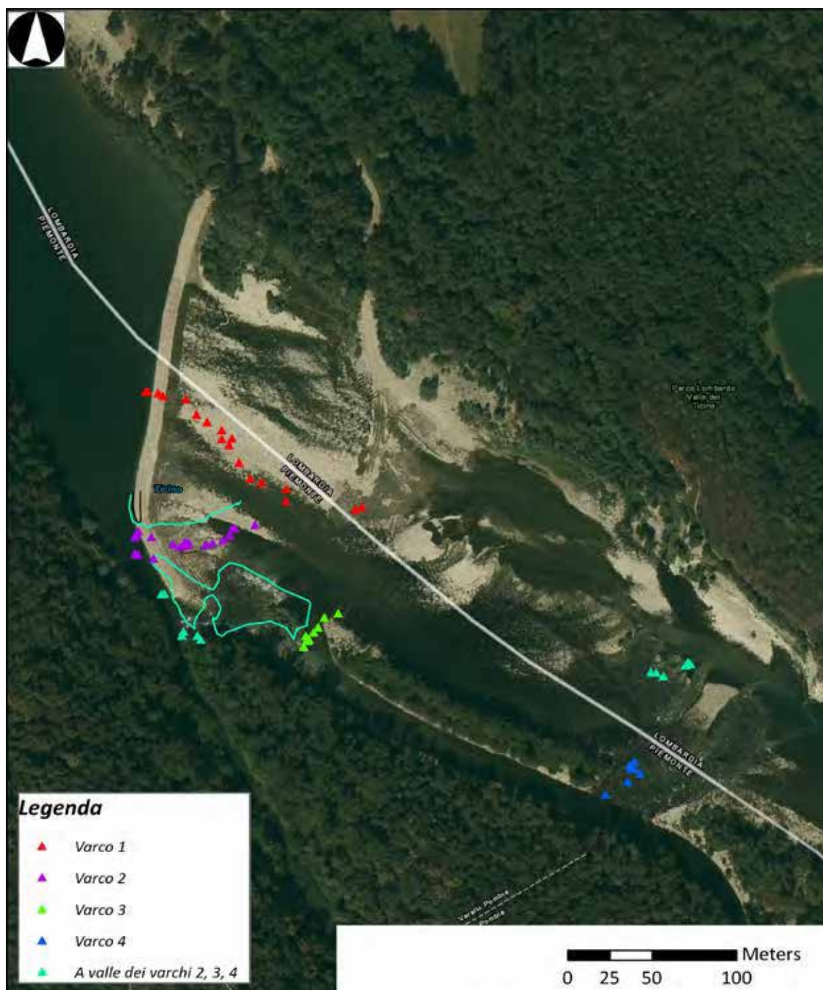
Figura 2.14: filarola a servizio delle rogge Novaresi - rilievo dei parametri idraulici
