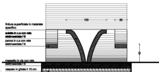
SEZ. B-B' modulo tipo: particolare costruttivo
