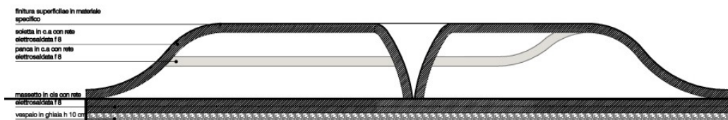
SEZ. A-A' modulo tipo: particolare costruttivo
